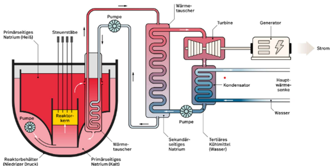
Abbildung 2: Schematische Darstellung eines Natriumgekühlten Schnellen Reaktors ( BASE - Alternative Reaktorkonzepte (bund.de) )
